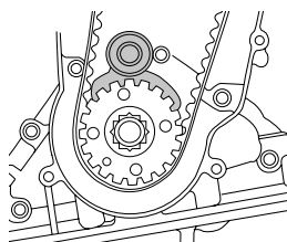
Фиксатор коленвала
