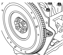
Фиксатор маховика
